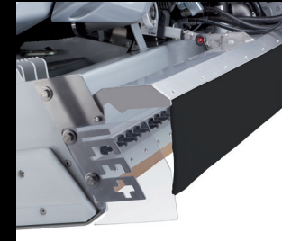
ICEplus Flexi Wassersprühsystem + automatischer Wischtuchheber
