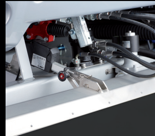
Wischtuchheber Automatisch
