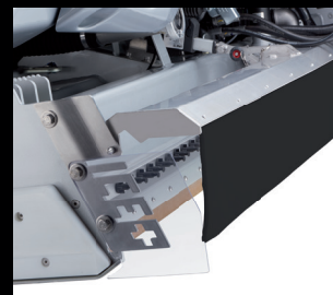
ICEplus Flexi 水喷洒系统 + 电动分水帘 挂板
