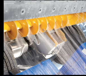
Kierukan pesulaitteisto vaakasuora
