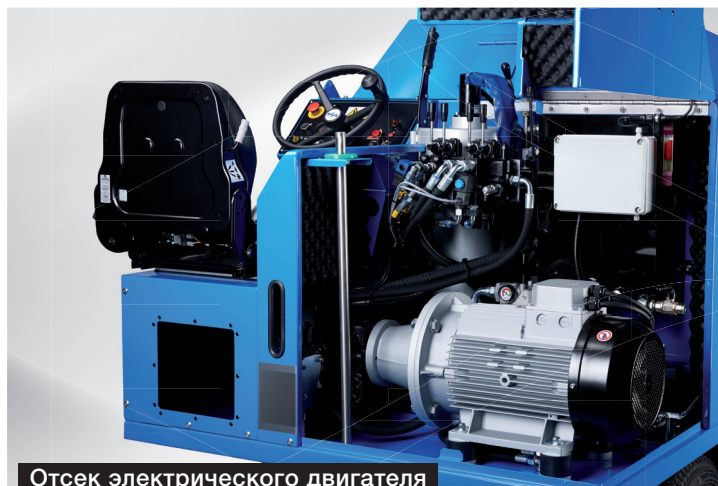
Отсек электрического двигателя
